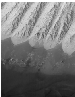
(d) Boundary (MGS MOC Image)
